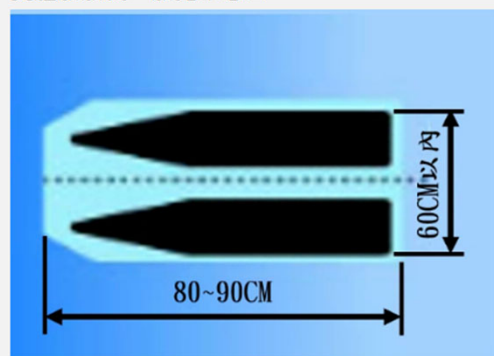
雙體船船長、船寬示意圖
